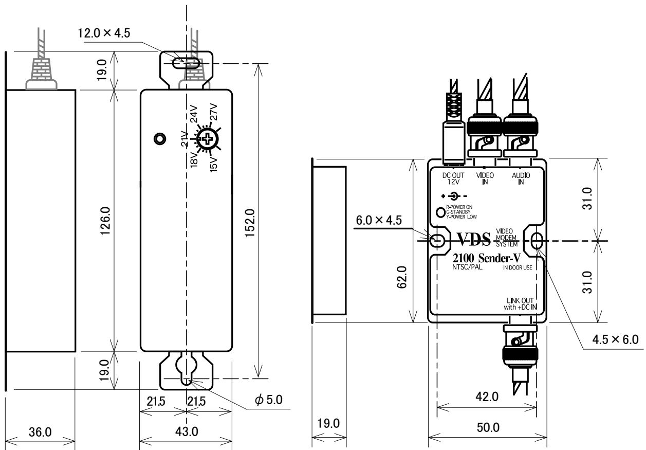
側面図
