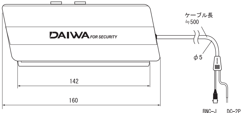
側面図
