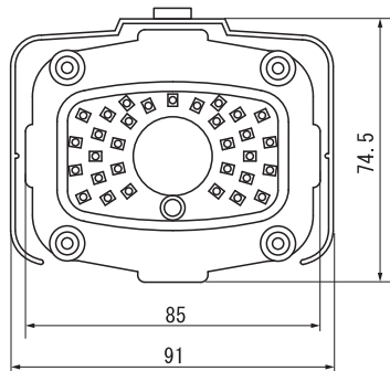
底面図
