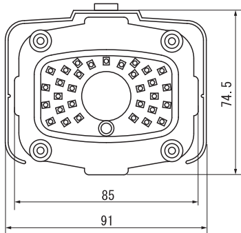
底面図
