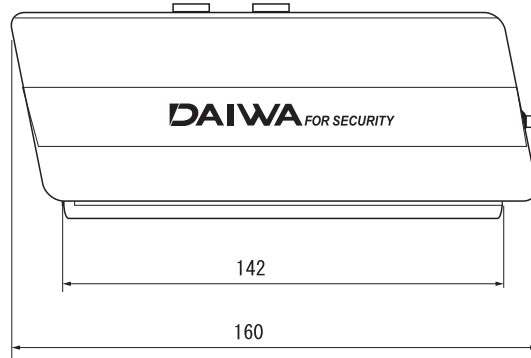
側面図
